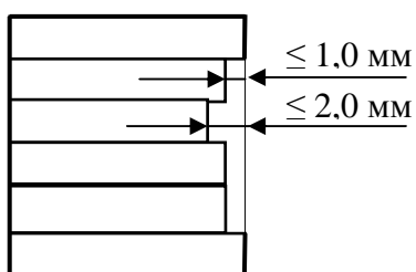
Рисунок 2 – Схема определения уступов ламелей
